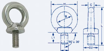
Golfare maschio ad occhio circolare in acciaio inox AISI316 con perno filettato
