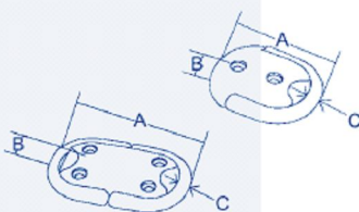
Base ovale con anelli, in acciaio inox AISI 316. Anelli con frizione antirollio.
