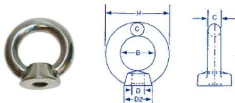
Golfare femmina ad occhio circolare in acciaio inox AISI 316 con foro filettato
